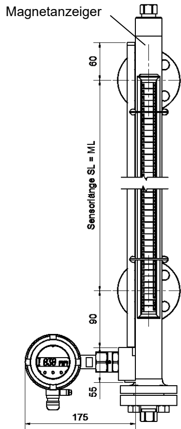
Abbildung 3: Füllstandmessung am Magnetanzeiger, Sensorkopf unten (Typ FFG-BP.20HXOD-D).
