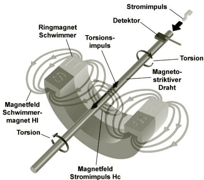
Abbildung 2: Wiedemann-Effekt.
